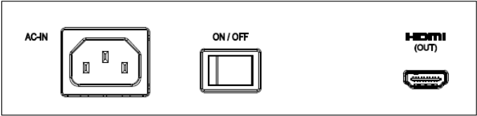
下侧I/O挡板 比例：5:1 丝印白色
